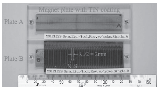
図6 試作したマイクロアンジュレーター用板状磁石 (提供：高エネルギー加速器研究機構 山本教授)
