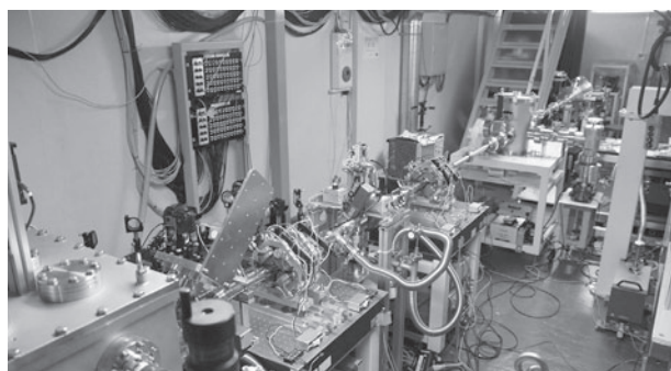
図5 レーザープラズマによる電子加速装置 （提供：大阪大学 細貝准教授）
