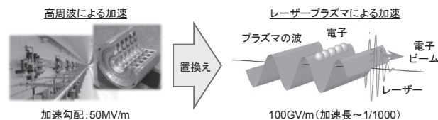
図2 高周波による電子加速とレーザープラズマによる加速
