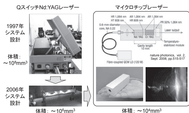
図3 レーザーピーニング用発振器の小型化
